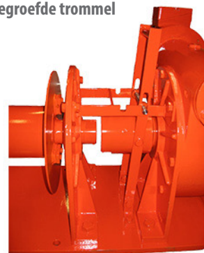
Vrijlooppkoppeling
