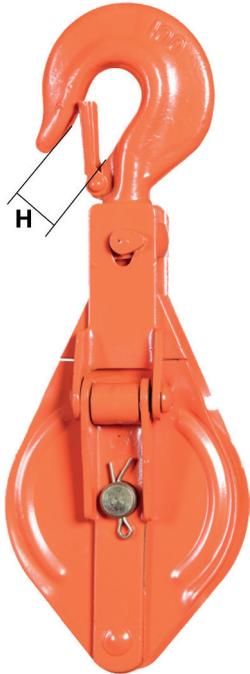
KBH1 met 1 staaldraadschijf
